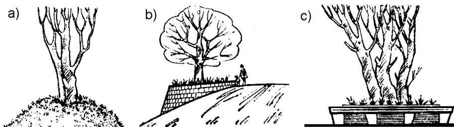
a) przekrój ogólny, b) szczegół wykopu, c) wstępna faza zabezpieczenia, wykonywana najlepiej rok przed właściwym wykopem Rys. 2. Zabezpieczenie drzew przy obniżeniu terenu, po wykonaniu wykopów (wg N.P. Ornatski: Drogi i ochrona przyrody, Transport 1982)
