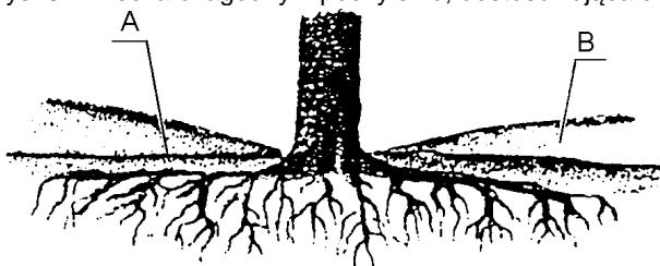
A - pierwotny poziom gruntu B - obsypka z lekkiej ziemi Rys. 4. Pień drzewa obsypany na wysokość 0,2 ÷ 0,5 m ze specjalnymi napowietrzającymi warstwami żwirowymi (wg [10])
