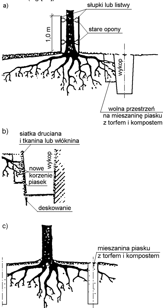
a) przekrój ogólny, b) szczegół wykopu, c) wstępna faza zabezpieczenia, wykonywana najlepiej rok przed właściwym wykopem Rys. 2. Zabezpieczenie drzew przy obniżeniu terenu, po wykonaniu wykopów (wg N.P. Ornatski: Drogi i ochrona przyrody, Transport 1982)
